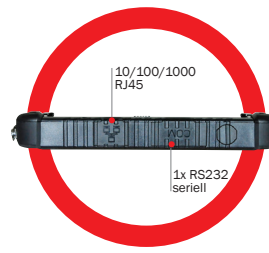
Seitenansicht links
