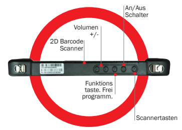
Seitenansicht oben
