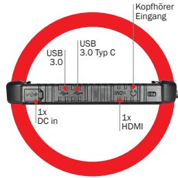
Seitenansicht rechts
